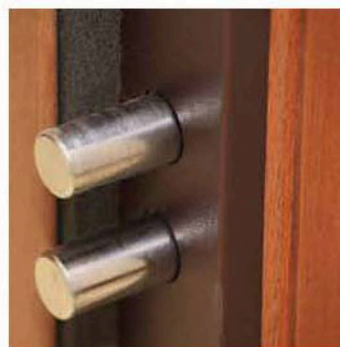
Particolare doppio deviatore
